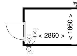
begane grond
